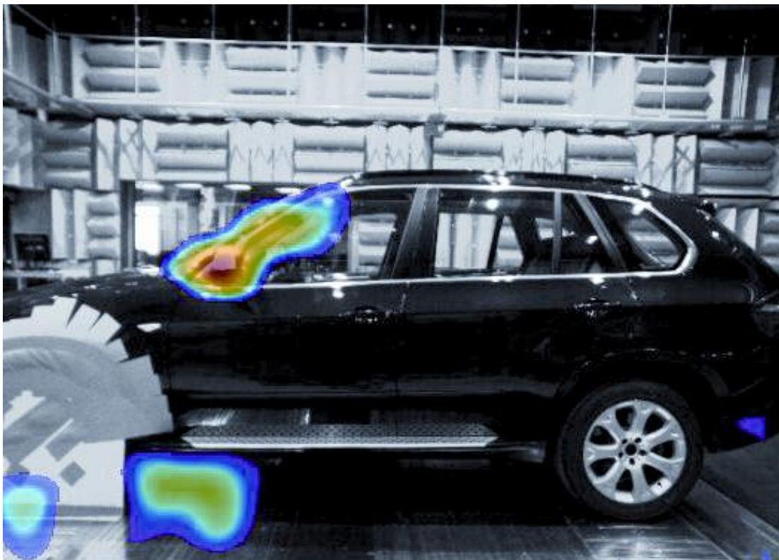
Rys.4. Samochód w tunelu aerodynamicznym
