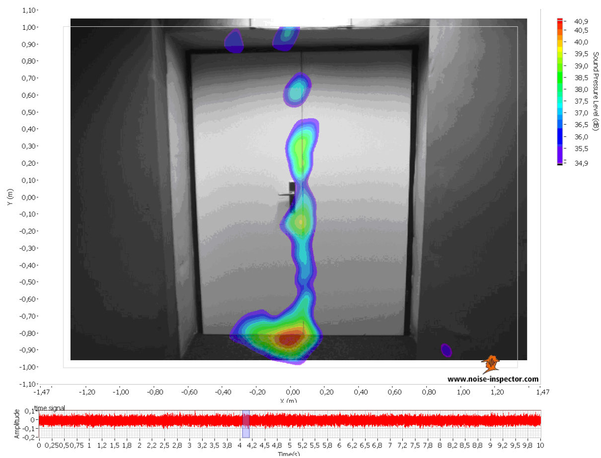
Rys.9. Drzwi
