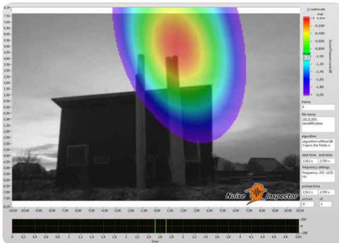
Rys.11. Hala przemysłowa
